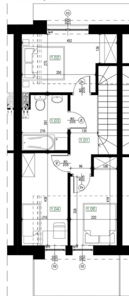
RZUT PIĘTRA
